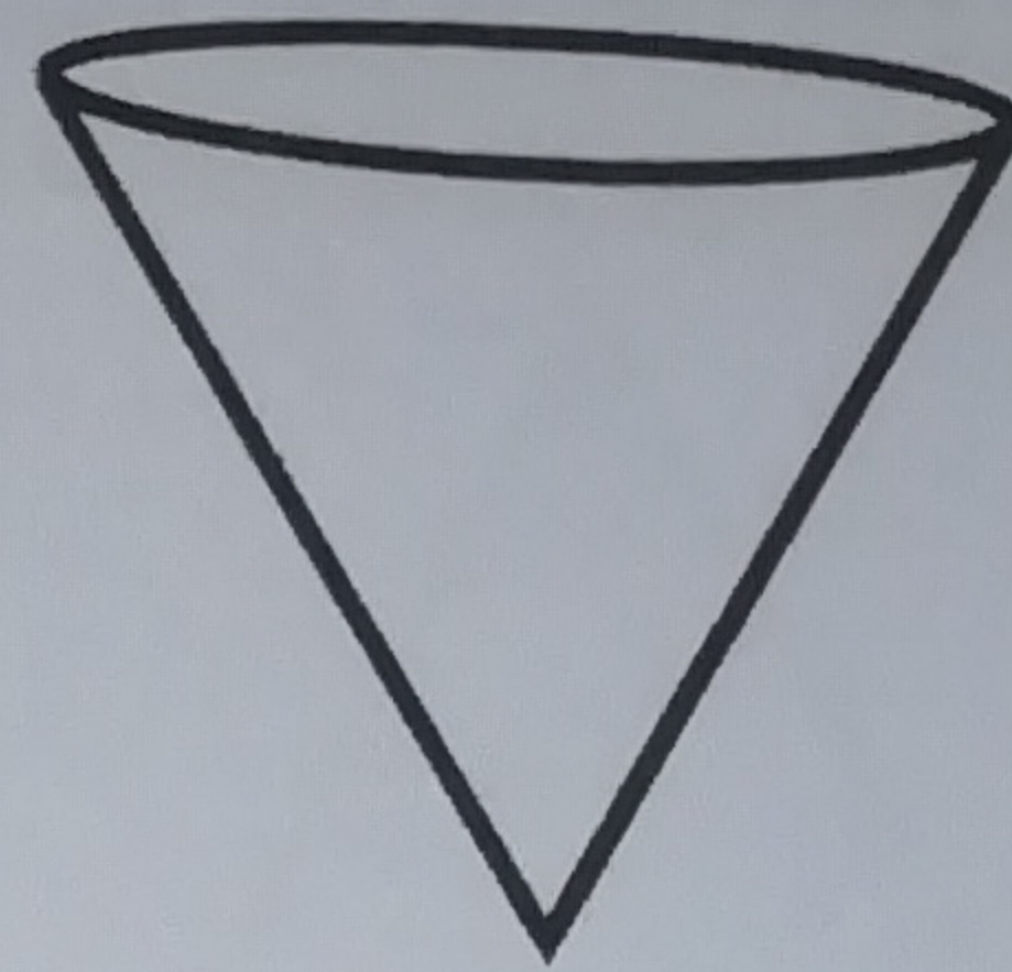
Cone
