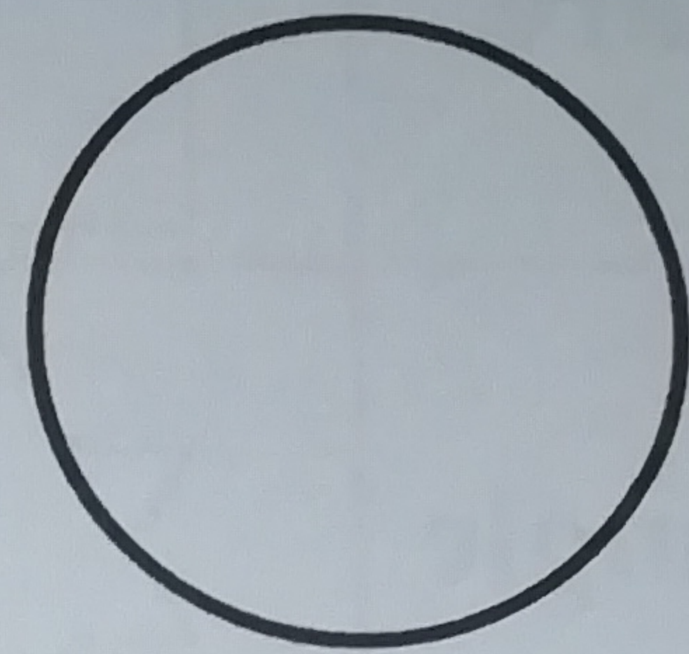
Circle
